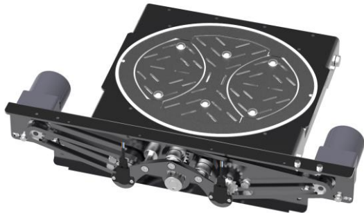
Drehrostmodul inkl. Drehroste und Motoren
